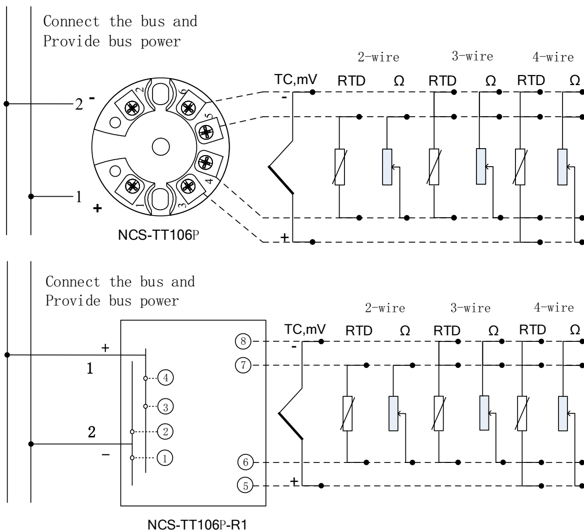
Figure.3 Wiring
